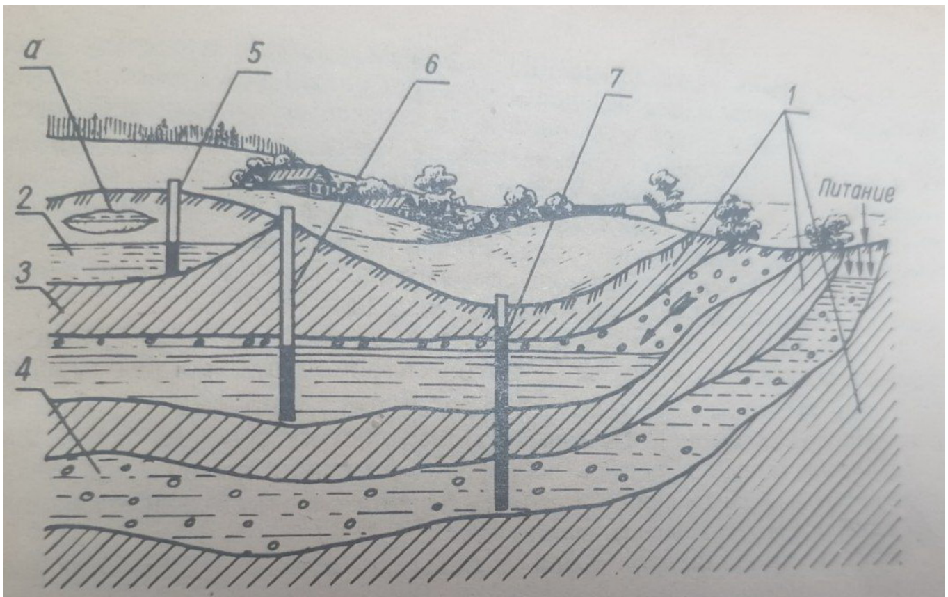
Рис. 1. Общая схема залегания подземных вод:
